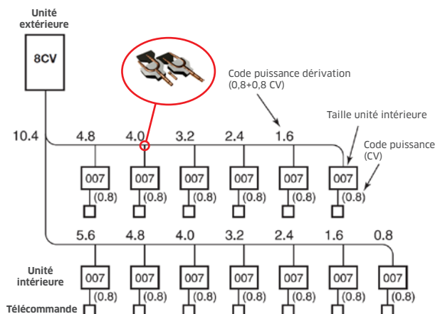
EXEMPLE DES LIAISONS ENTRE DÉRIVATIONS (SMMS u ) :
